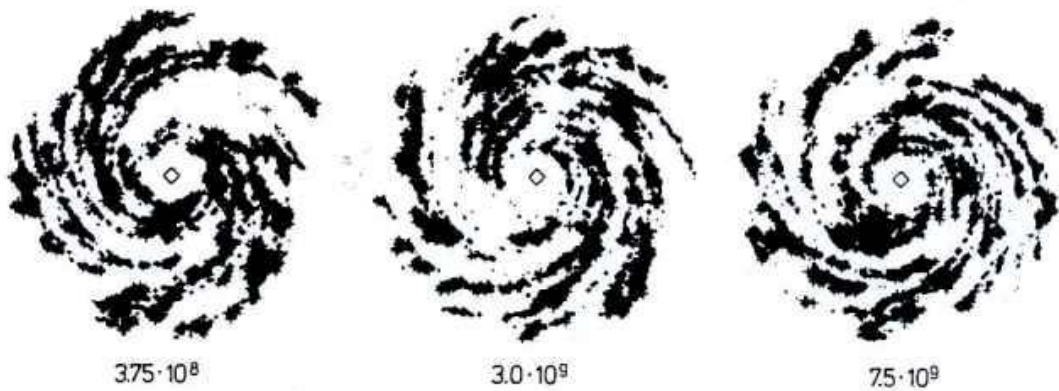
Abb. V.22 Entwicklung der Struktur einer Modell-Galaxie. Es wurde die Rotationskurve von M81 zugrunde gelegt. Die beigefügten Zahlen beziehen sich auf die seit dem Beginn der Rechnung verfllossene Zeit in Jahren. (Nach H. Gerola und P.E. Seiden).
